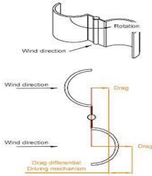
Şekil 2. Rotorun Profil Görünümü
